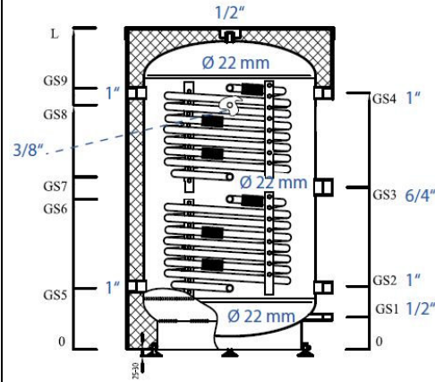
Speicherschema 200l, 2 WT
