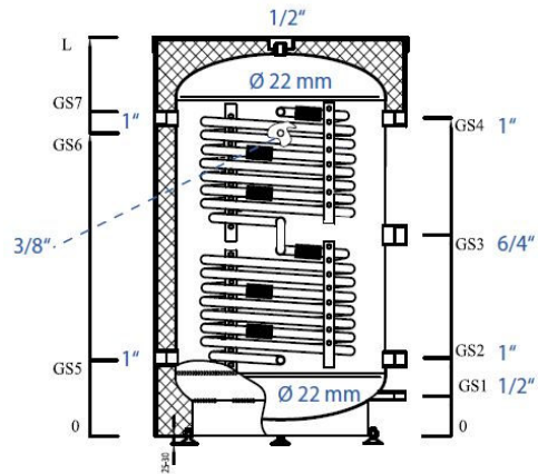
Speicherschema 200l, 2 WT verbunden zu 1 WT
